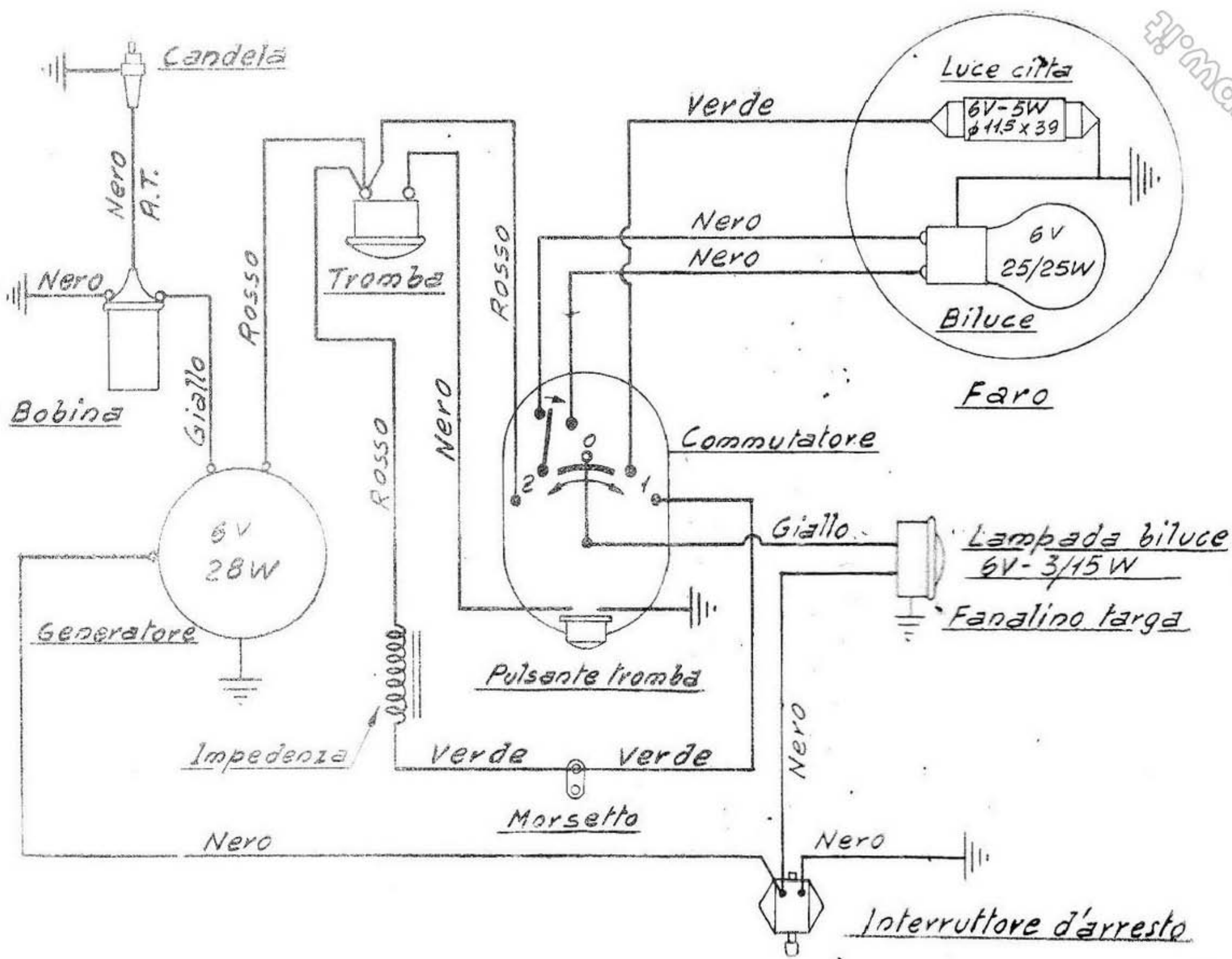
Fig. 19 - Schema impianto elettrico
